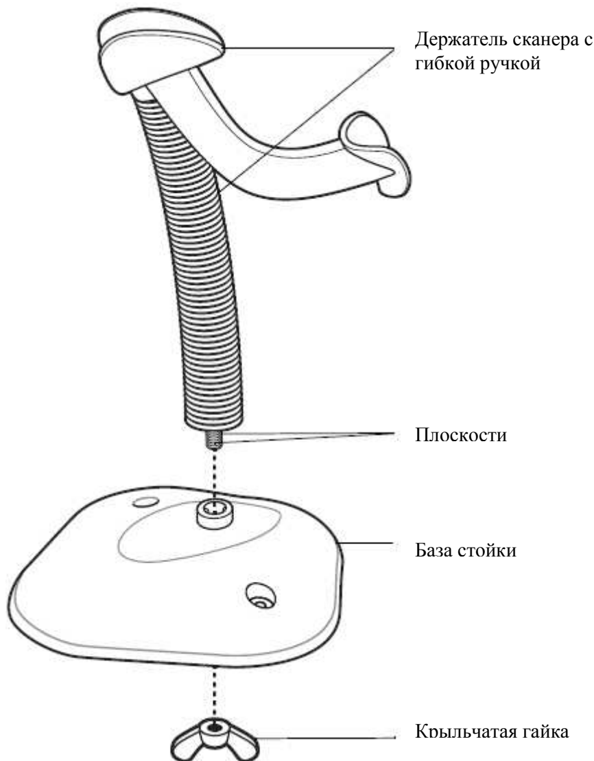
Рисунок 2-2 Сборка стойки
