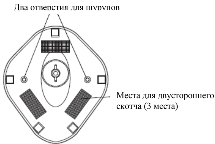
Рисунок 2-3 Крепление стойки
