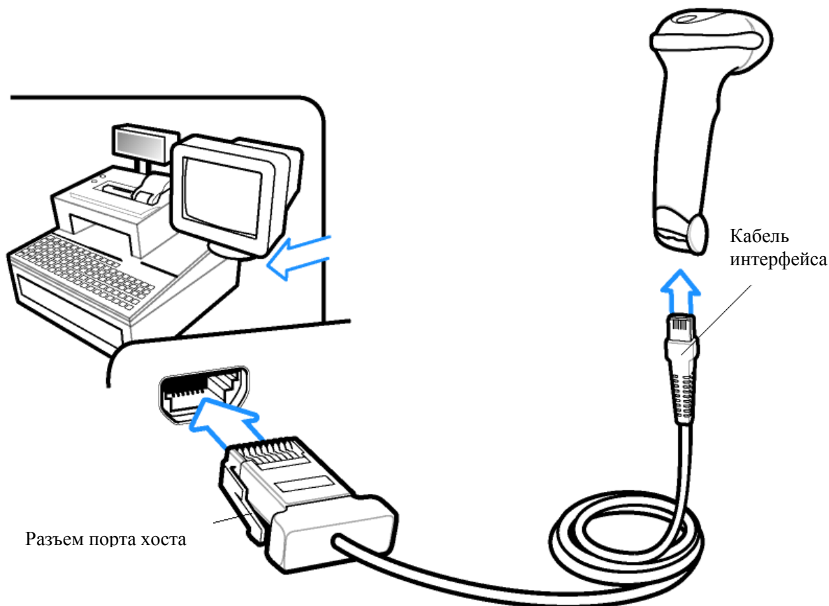
Рисунок 7-1 Прямое подключение IBM
