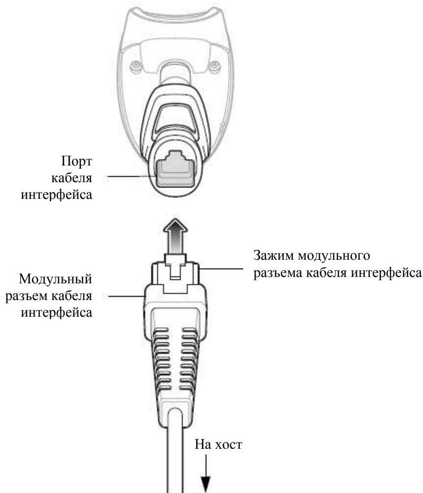
Рисунок 1-2 Установка кабеля
