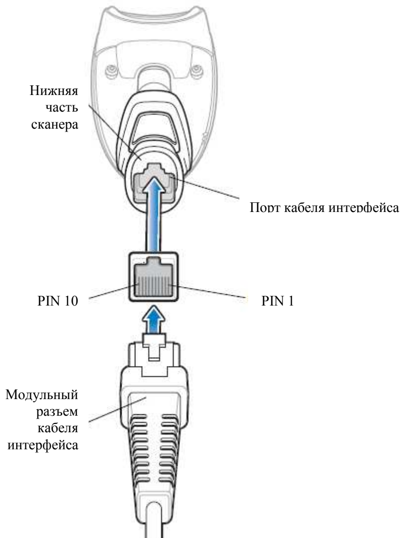
Рисунок 3-1 Выводы кабеля цифрового сканера
