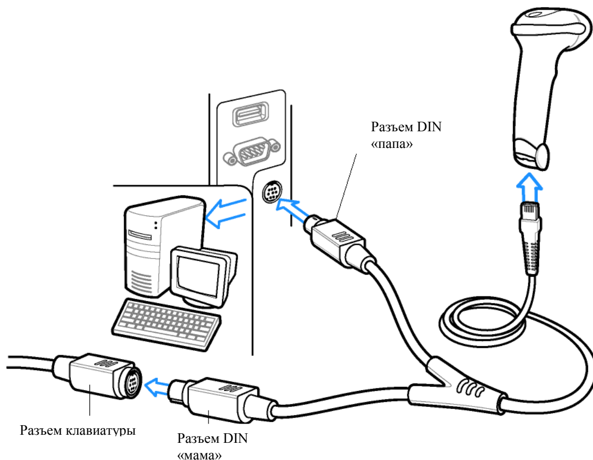
Рисунок 8-1 Подключение Keyboard Wedge с Y-образным кабелем
