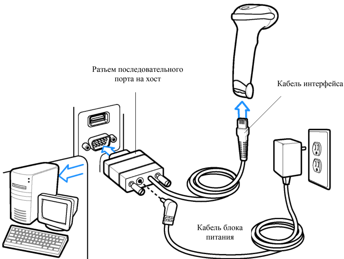
Рисунок 6-1 Прямое подключение RS-232
